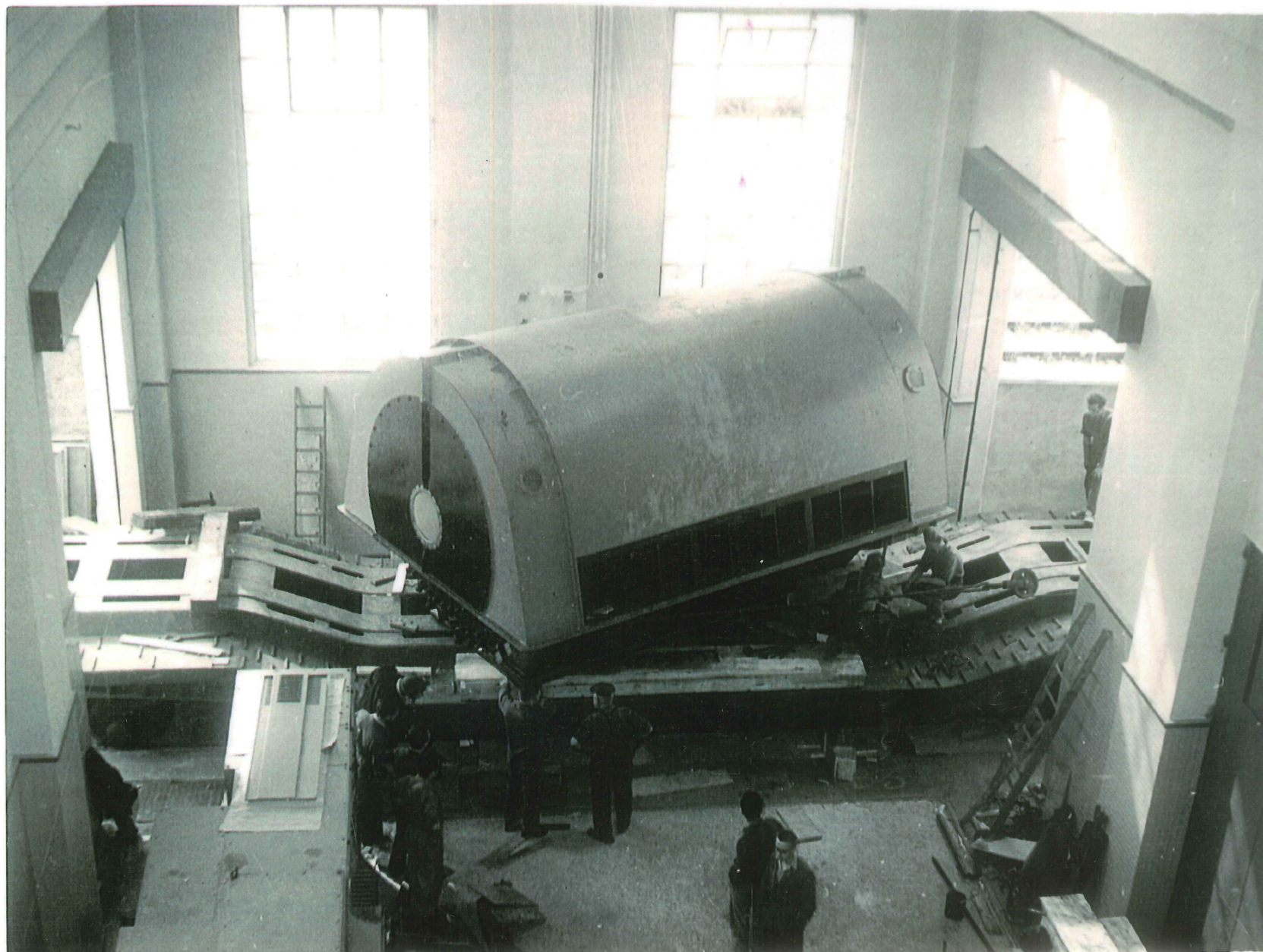
Livraison du stator de l'alternateur JEUMONT
