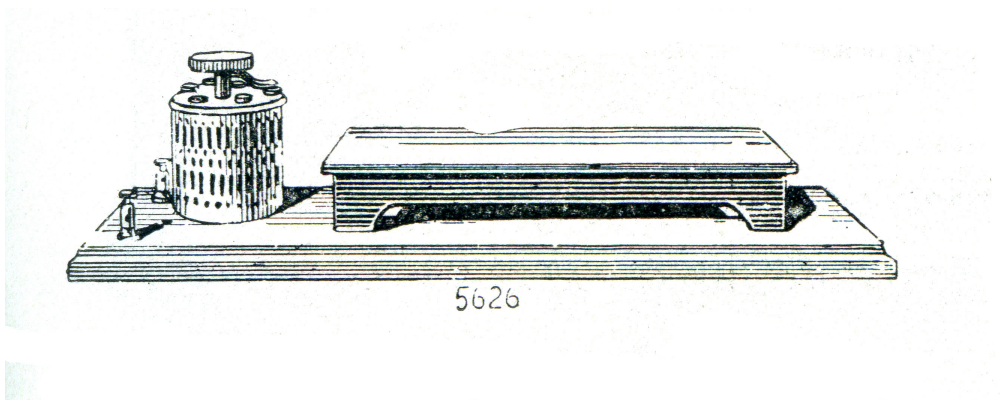
5626 Platine chauffante électrique du Professeur Policard , à 6 allures de chauffe. (Voltage du courant : 110 ou 220 v., à spécifier à la commande.)
