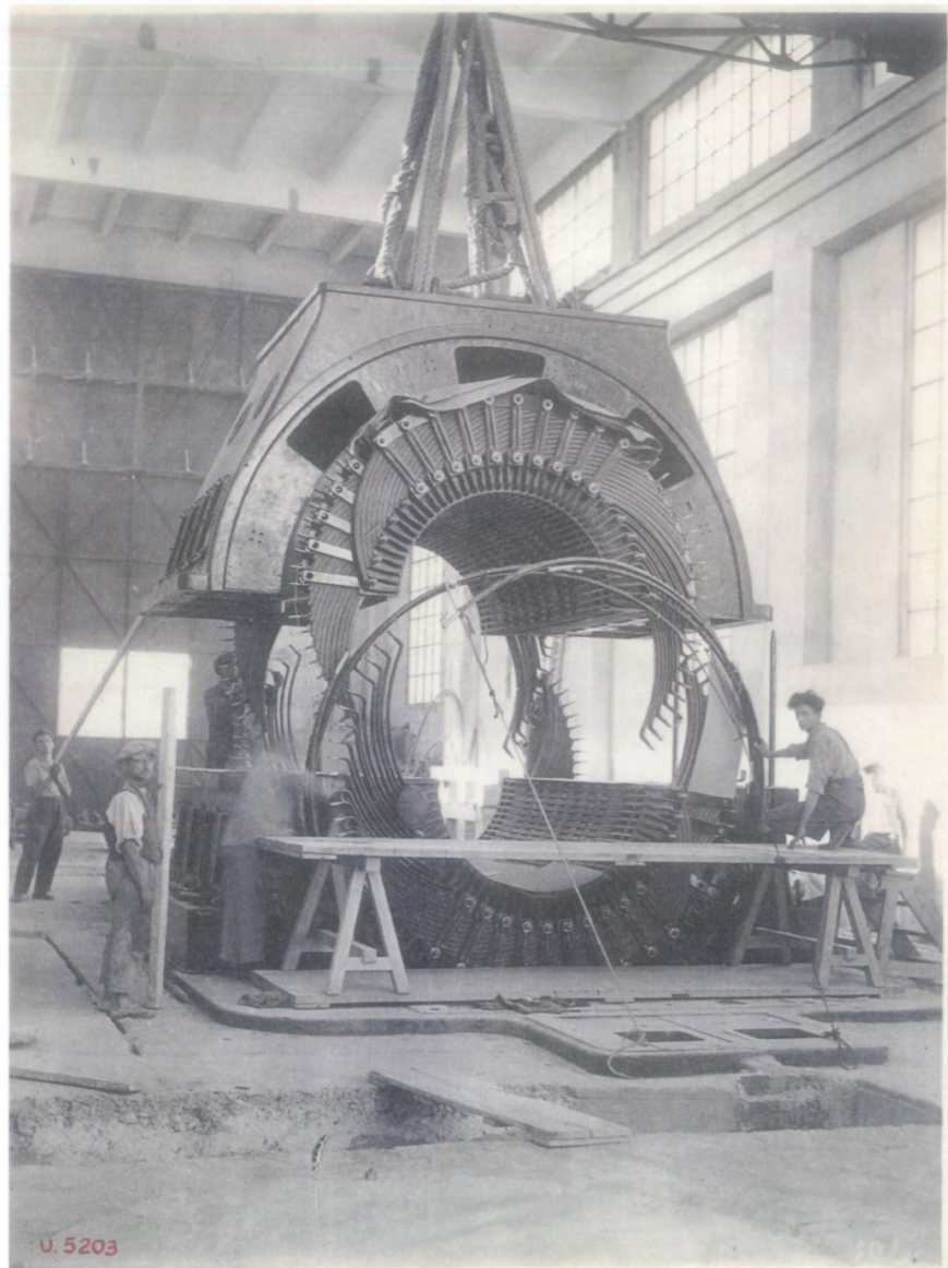
Assemblage du stator de la 600 MVA (1928)
