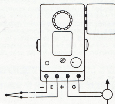
Fig 4 - GALVANOMETRE EXTERIEUR
