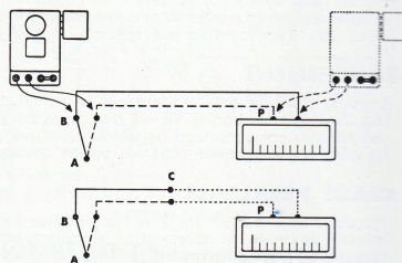
Fig 5 - CONTROLE D'UN PYROMETRE EN SERVICE
