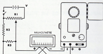
Fig 6 - ETALONNAGE D'UN MILLIVOLTMETRE
