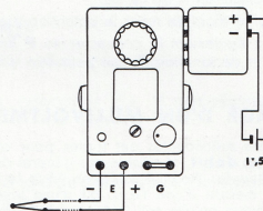
Fig 3 - PILE SEPARÉE
