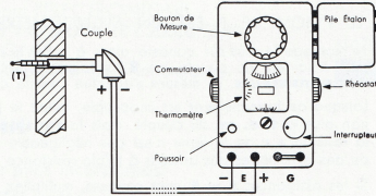
Fig 2 - MESURE D'UNE TEMPÉRATURE
